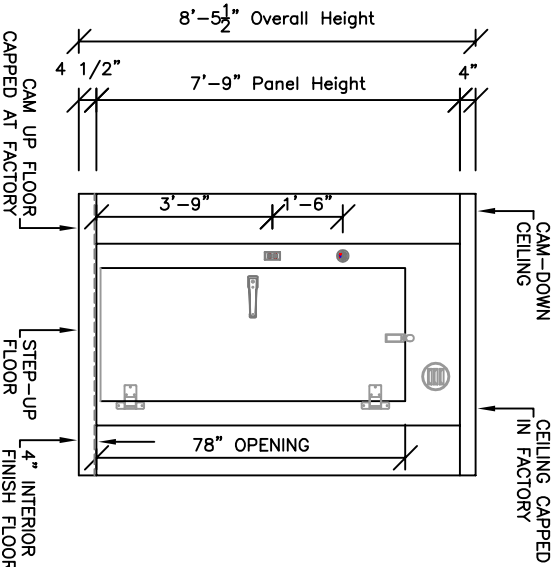
ELEVATION
